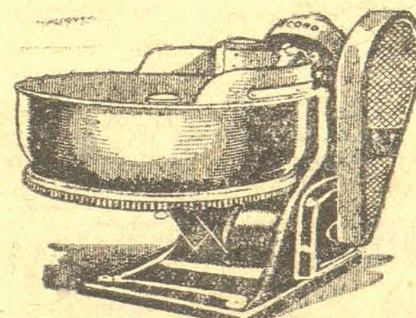
AMASSADEIRAS "RECORD" COM CAPACIDADE PARA 30, 70, 150, 300 E 400 KGS.
