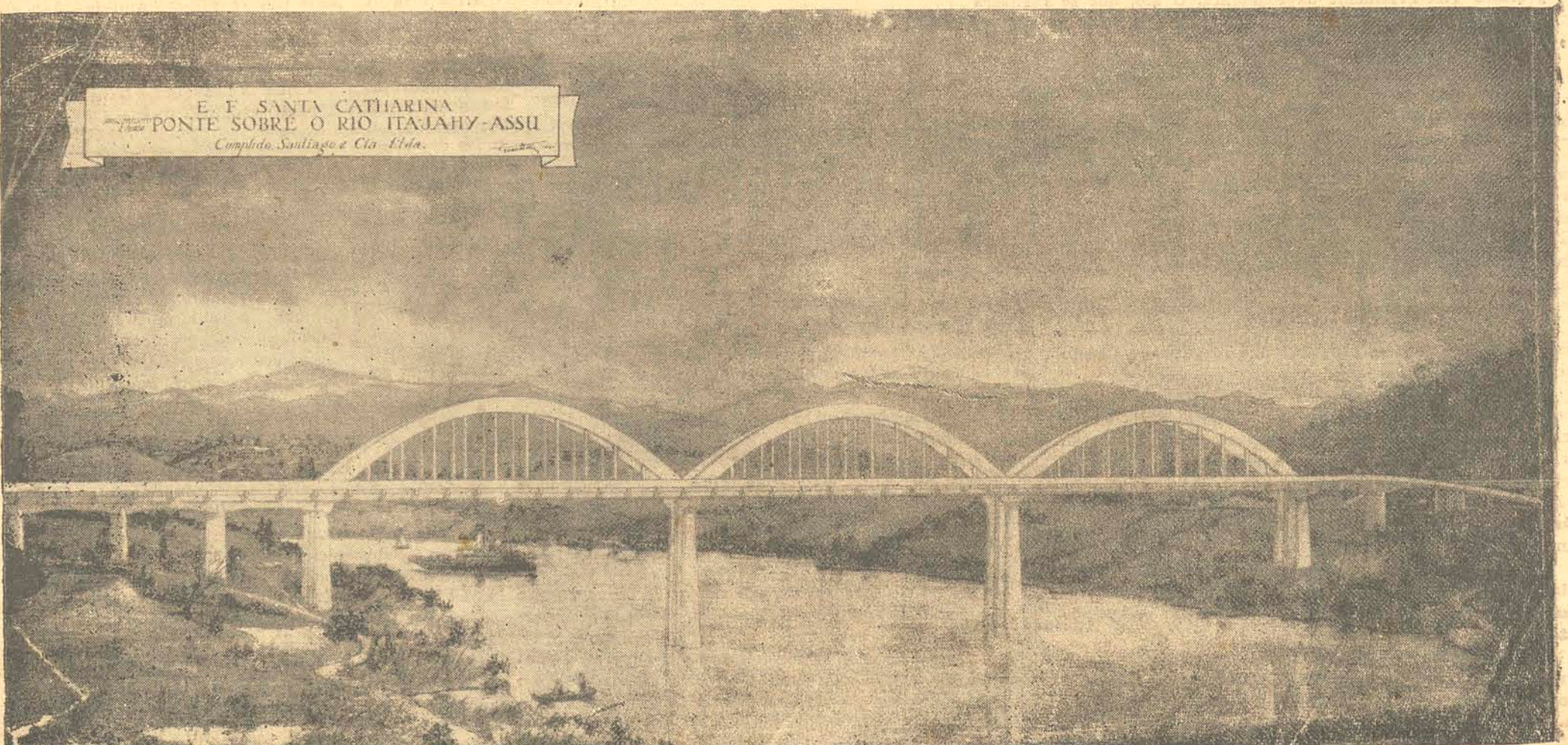
Ponte sobre o rio Itajaí-Açu, em construção pela firma Cumplido, Santiago & Cia. Ltda. (ante-projeto)
