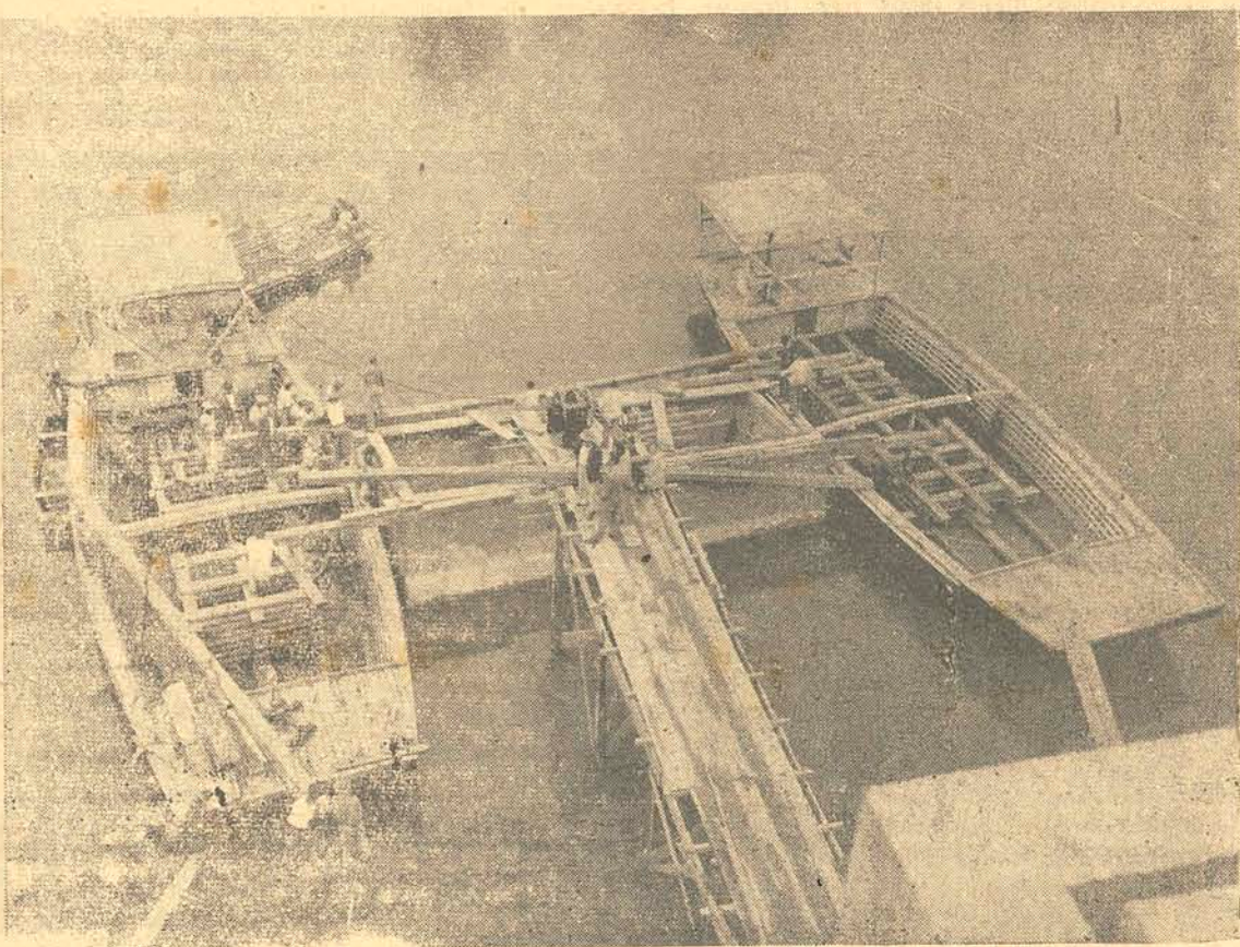
Caixão de concreto armado, flutuante, entre batelões
