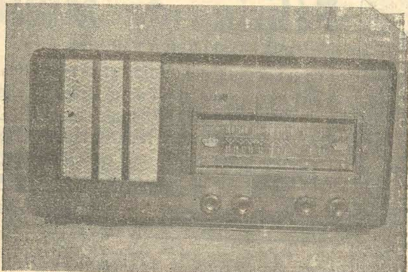
Para Bateria — 6 volts — 2 faixas — Alto-falante 6 1/2 polegadas. Consumo 2 ampers por hora.
