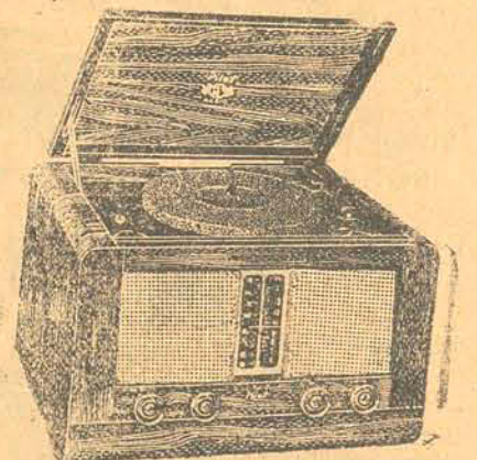
RADIO-VITROLA — Modelo PB-4 — 6 Valvulas — Ondas Curtas e Longas. — Transformador Universal. — Alto-falante 6” polegadas. — Em artístico movel de Imbuia.
