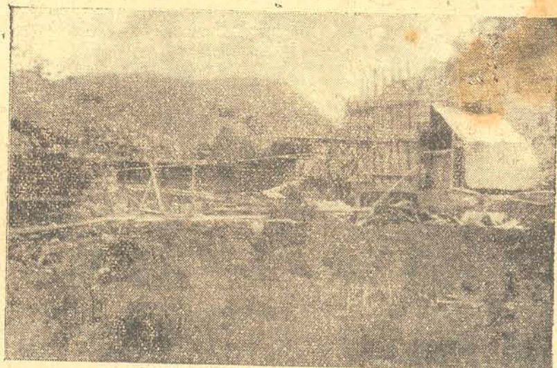
Aspecto da barragem do 8º Salto
