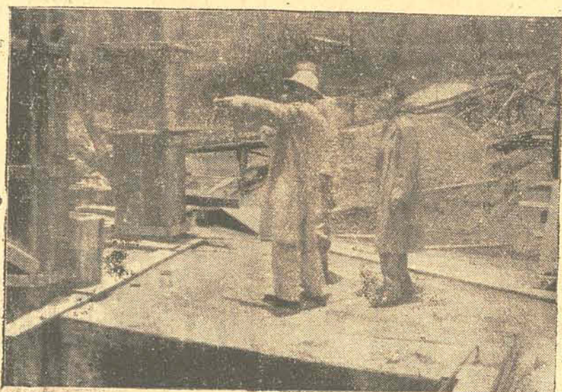
Aspecto da visita às obras de barragem no rio Bracinho, cujas obras foram iniciadas em 16 de outubro de 1944, 13 quilômetros de rodagem, 12 quilômetros de linha de alta tensão, alojamento, escritório, armazem, padaria e a construção da barragem do 8º Salto
