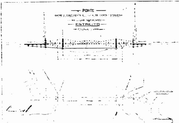
Projecto de ponte apresentado ao Governo do Estado
