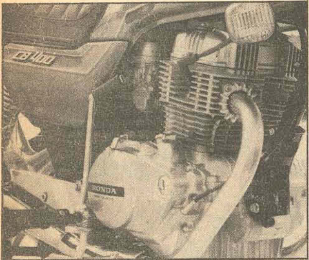
O motor de 395 cc da Honda CB-400 é de concepção moderna, com seus dois cilindros dispostos em "Parallel-Twin" e válvulas no cabeçote, que o tornam o motor mais avançado da indústria nacional de motos.
