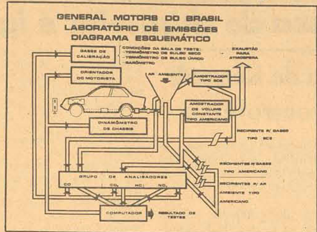
Do dinamômetro, os dados obtidos são remetidos aos computadores e analisados pelos engenheiros.
