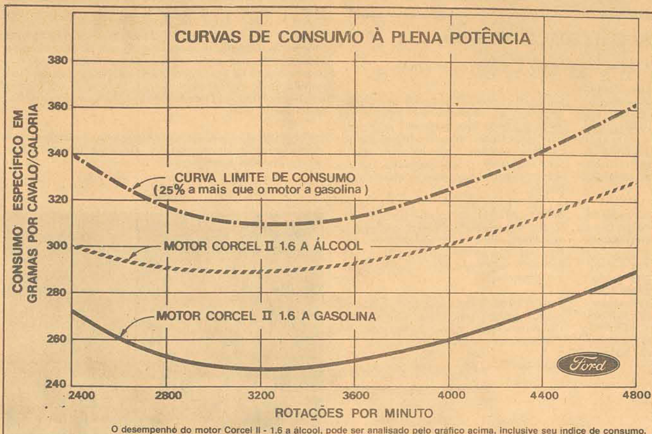
O desempenho do motor Corcel II - 1.6 a álcool, pode ser analisado pelo gráfico acima, inclusive seu índice de consumo.
