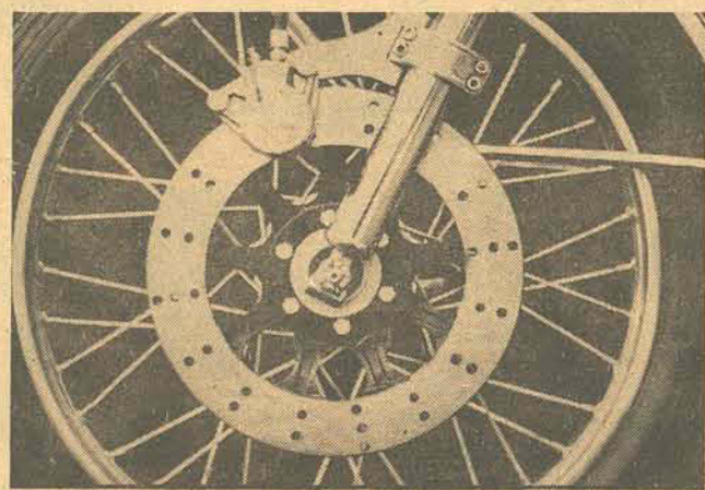
Ralação em três diâmetros, disco em liga especial e furação dimensionada para evitar o "squeal", dão maior segurança ao hidráulico Doppler.
