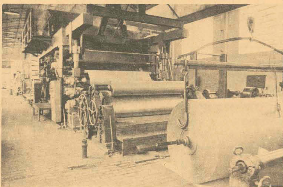
...que utiliza resíduos de serrarias, aparas e pasta mecânica para produzir papel em suas máquinas e caldeiras alimentadas a lenha...
