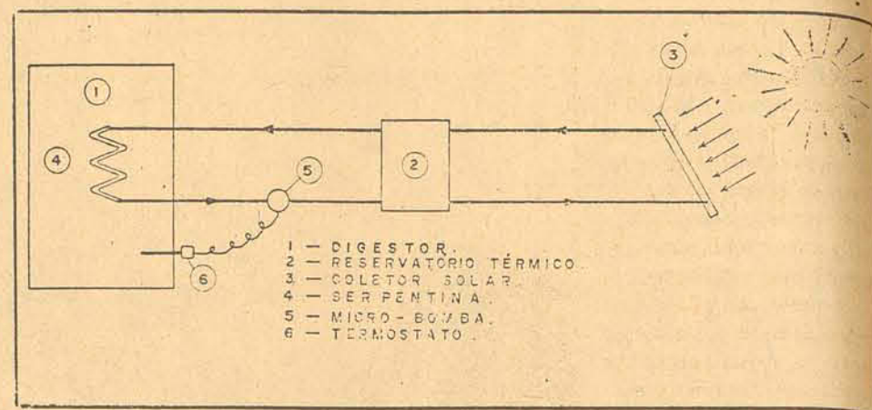
Esquema para utilização de energia solar visando aquecer a biomassa.
