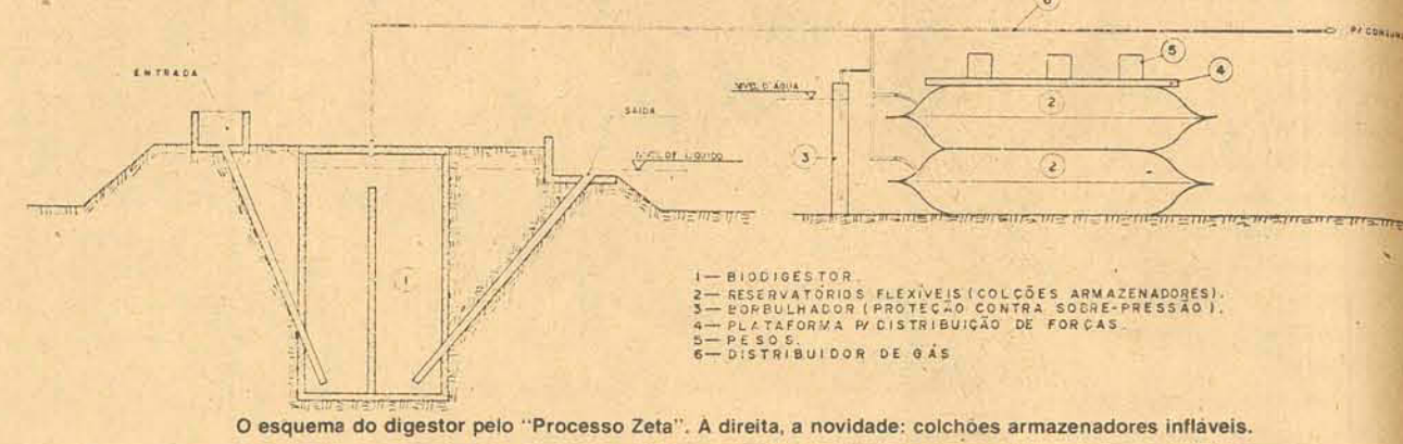
O esquema do digestor pelo "Processo Zeta". A direita, a novidade: colchões armazenadores infláveis.
