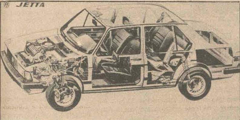
O Jetta, em corte, mostra o seu amplo espaço interno, inclusive do porta-malas, bem como, alguns detalhes de sua mecânica, como o motor transversal, refrigerado a água.
