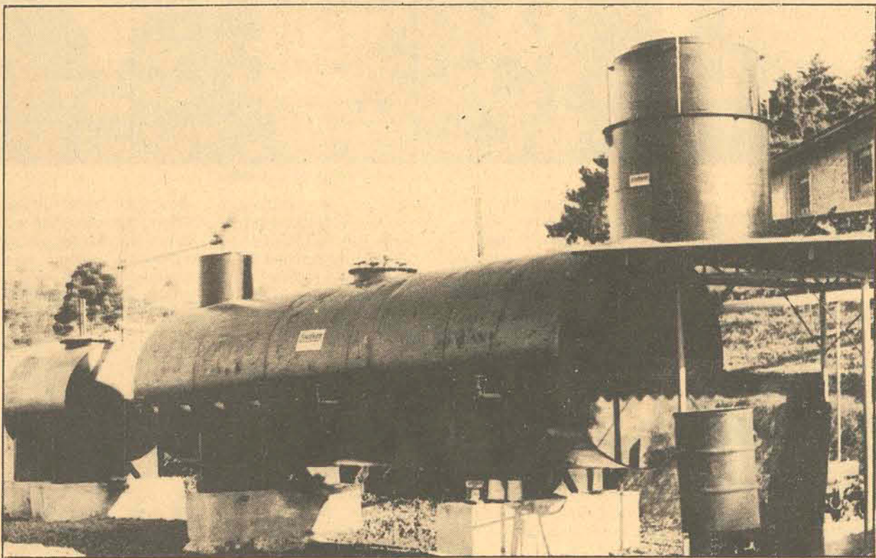
A unidade de biogás instalada na localidade de São Braz, em Joaçaba.
