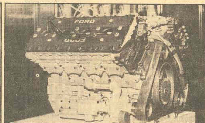
O motor Ford-Cosworth do Copersucar F-6, tem 8 cilindros em "V", 2.993 cc e alcança os 495 HP a 10.500 rpm.
