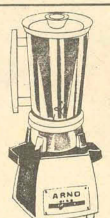
LIQUIDIFICADOR ARNO LR - 3 velocidades reguláveis com interruptor, sobretampa servindo como medidor, jarra térmica com alça.
