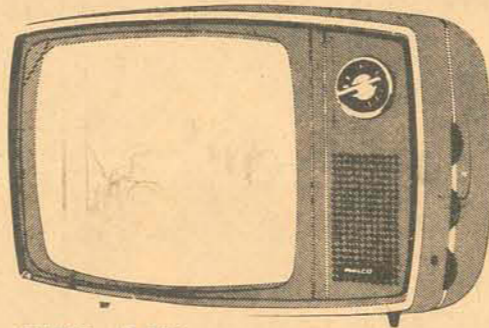
TV Philco B-265 Portátil. Tela de 31 cm (12") Preto e branco. Totalmente transistorizado. Funciona em 110 e 220 V e em bateria de 12 volts. Alça embutida na parte traseira do aparelho. Com regulador automático de voltagem.
