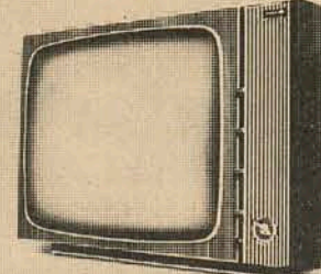
Modelo B-140, Preto e Branco, 61 cm (24 polegadas). Totalmente transistorizado. Controles lineares deslizantes. Móvel em madeira de lei. Funciona em 110, 127 e 220 volts. Imagem inabalável, garantida pelo DS-388.
