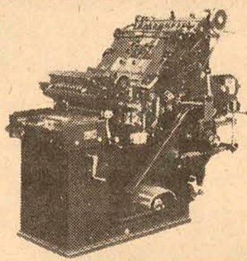
Impressora Catu 380 - interior Interior da rama 275 x 380 mm velocidade máxima 4.200 fls. p/hora.
