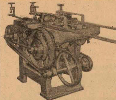
FURADEIRA P/MONTANTES DE VENEZIANAS
