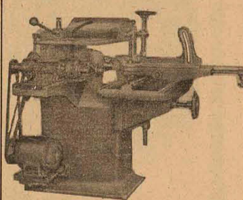
RESPIGADEIRA SEMI-AUTOMÁTICA
