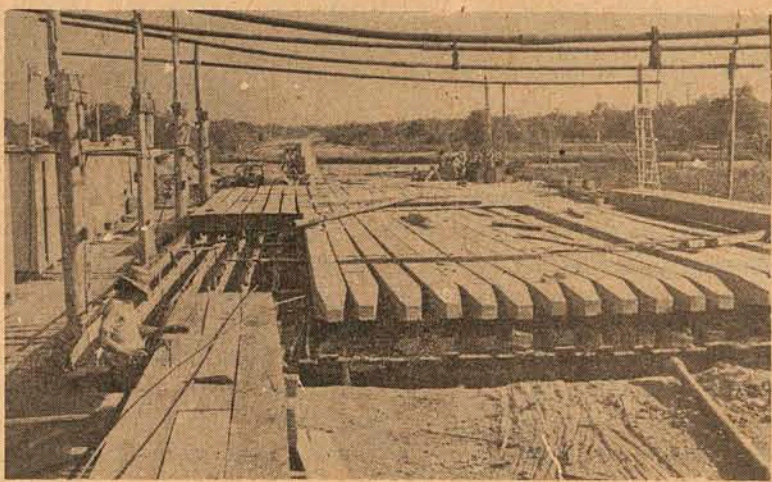
A velha ponte oferece uma silhueta medieval.
