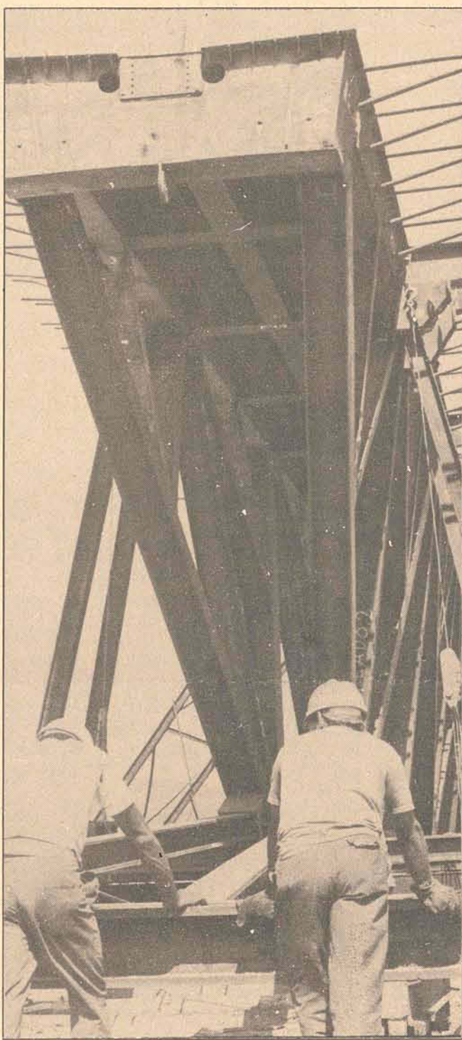
A gigantesca treliça se interpõe entre os pilares 3 e 4.
