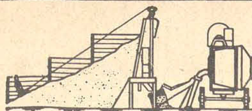
Usina de concreto Donar e Pá Arrastadora Donar
