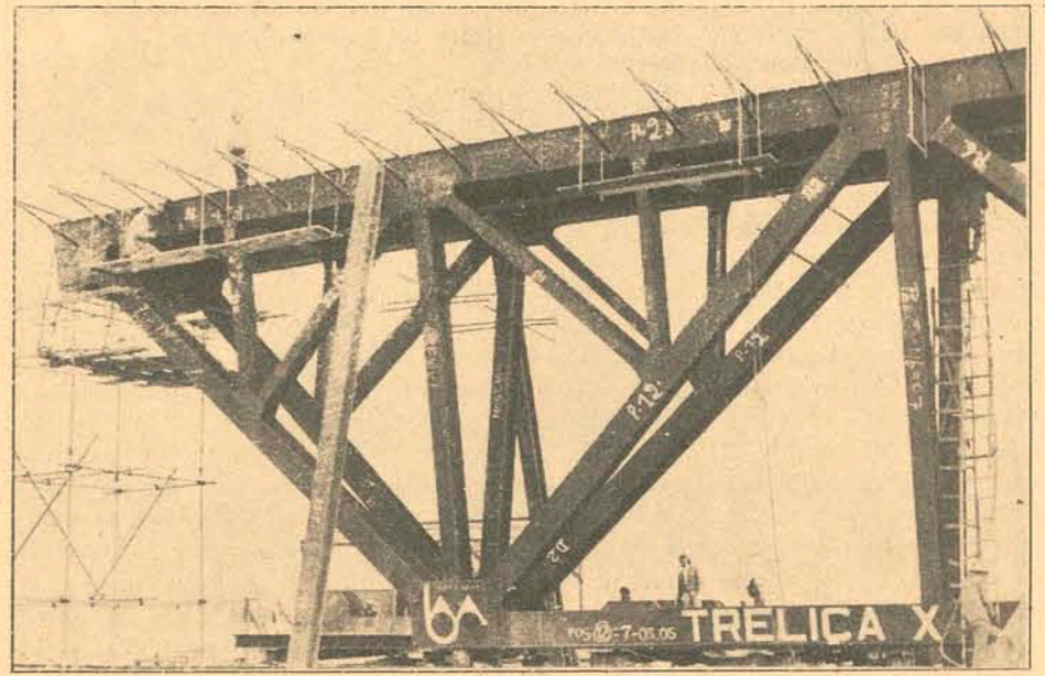
No canteiro de obras estão as imensas treliças de aço, com 160m.
