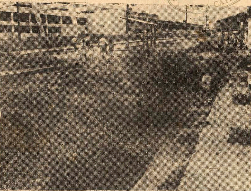
Com a finalidade de evitar o deslocamento dos paralelepípedos logo após o término dos serviços de calçamento da Avenida Mauro Ramos, a Prefeitura Municipal de Florianópolis, conforme mostra a foto, está cuidando da construção de valas e bueiros para o escoamento das águas pluviais.
