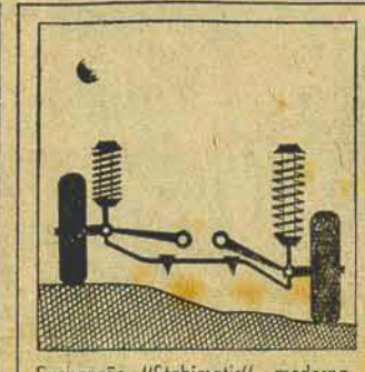
Suspensão "Stabilomatic", moderna; incomparável aderência nas curvas e em altas velocidades. Absorve toda a tríplicação - maior obediência em marcha; maior estabilidade!
