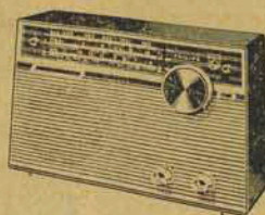
R3 RO 67 Radio receptor de mesa, com 7 transistores e 2 diodos, 3 faixas de ondas. Alimentado com 4 pilhas comuns.
