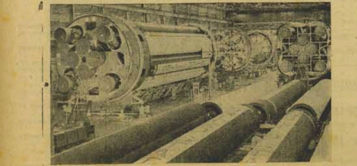
Vista da linha de montagem do Centro Marshall. Aero Espacial de Huntsville em Alabama mostrando as partes do Saturno I em várias etapas de montagem. O Saturno que deverá desenvolver 600 mil quilos de empuxo, está sendo fabricado para ser utilizado no programa Apollo de astronautas tripuladas, tendo obtido pleno êxito em quatro lançamentos experimentais já efetuados.
