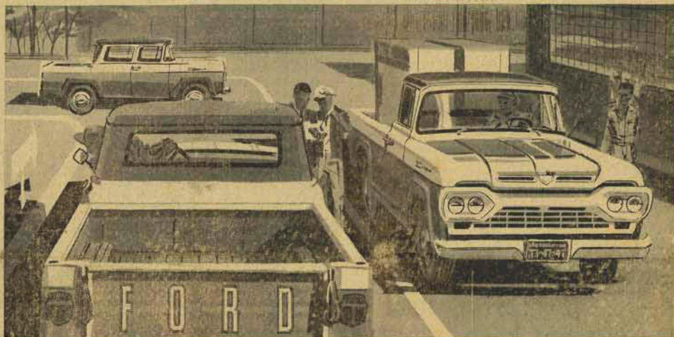
• SUPER FORD F-100 — Camioneta com o conforto, estilo e desempenho dos modernos carros de passeio: cabina espaçosa, pára-brisa panorâmico, alavanca de câmbio na direção, assento e encosto de espuma de borracha. Fácil de manobrar, ágil no trânsito, ideal para entregas urbanas. Capacidade de carga: 930 kg. Motor: V-8, de 167 H.P. Distância entre eixos: 2,80 m.
