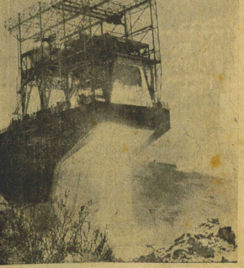
MOTOR SUPER-ESPACIAL — Línguas de fogo saem da câmara de empuzo durante o teste de estática, a que foi submetido o motor F-1, na Base de Força Aérea de Edwards, Califórnia. O motor super-espacial, destinado a produzir um empuzo de 680 mil quilos, será usado no foguete Nova durante os primeiros voos pilotados a Lua. Otto dos gigantes motores F-1 integrando a primeira etapa do veículo lunar.
