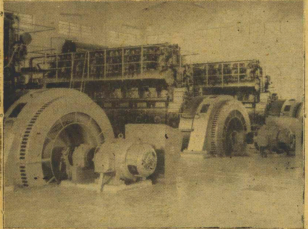
USINA DIESEL ELÉTRICA DE 3150 KVA — VENDENDO-SE EM CONJUNTO OS TRÊS GRUPOS GERADORES MARCA DEUTZ — GARBE — LAHMEYER.
