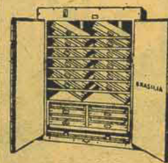
"BRASILIA" Incubadora elétrica para 2.400 ovos
