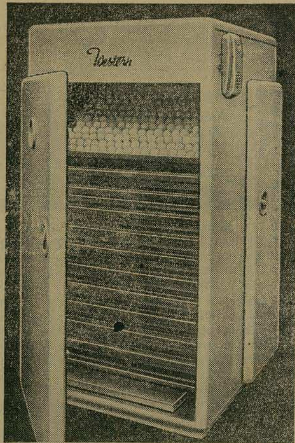
NOVA INCUBADORA — Incubadora Western, recentemente exibida em Londres. Neste aparelho, os ovos são mudados de posição cada hora. A operação é totalmente automática, realizada por um motor de uma fração de cavalo, controlado por um relógio que se regula à vontade — BRITISH NEWS SERVICE
