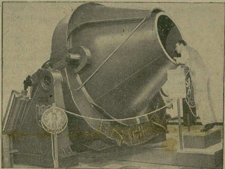
NOVO MISTURADOR DE CONCRETO — Giganteco misturador de concreto, feito pela firma Winget, de Rochester (Inglaterra), e capaz de fornecer 3 jardas cúbicas de concreto em cada operação BRITISH NEWS SERVICE
