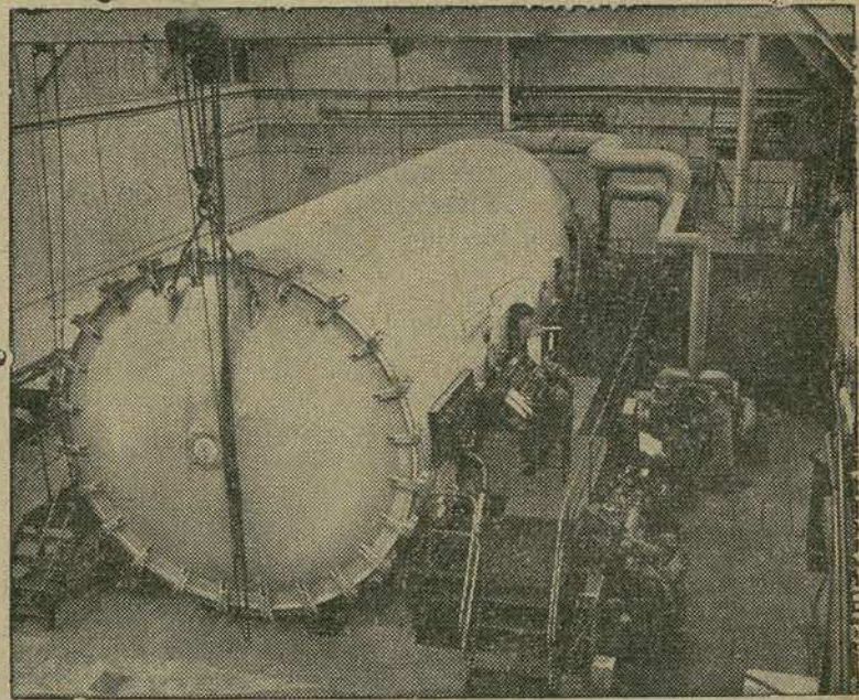
PARA OS AVIÕES DO FUTURO — A De Havilland Aircraft Co. Ltd., fabricantes dos famosos aviões a jato do mesmo nome, acaba de construir uma nova câmara de altitude, a fim de facilitar as pesquisas sobre o uso de equipamento aeronáutico na estratosfera. — BRITISH NEWS SERVICE
