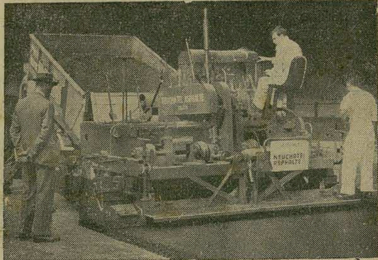
CONSTRUTOR DE ESTRADAS — A indústria britânica acaba de lançar um novo aparelho, o Barber-Greene Finisher, capaz de construir o leito de uma estrada ao ritmo de 2,5m. a 13, por minuto, conforme a espessura e largura da camada de concreto ou material asfáltico BRITISH NEWS SERVICE
