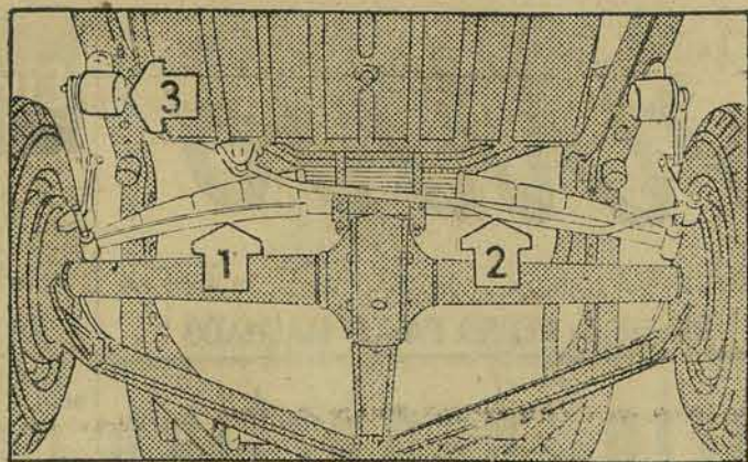
Novas molas, mais longas e com maior número de folhas (1). Novos estabilizadores laterais (2). Novos amortecedores hidráulicos de dupla ação (3).
