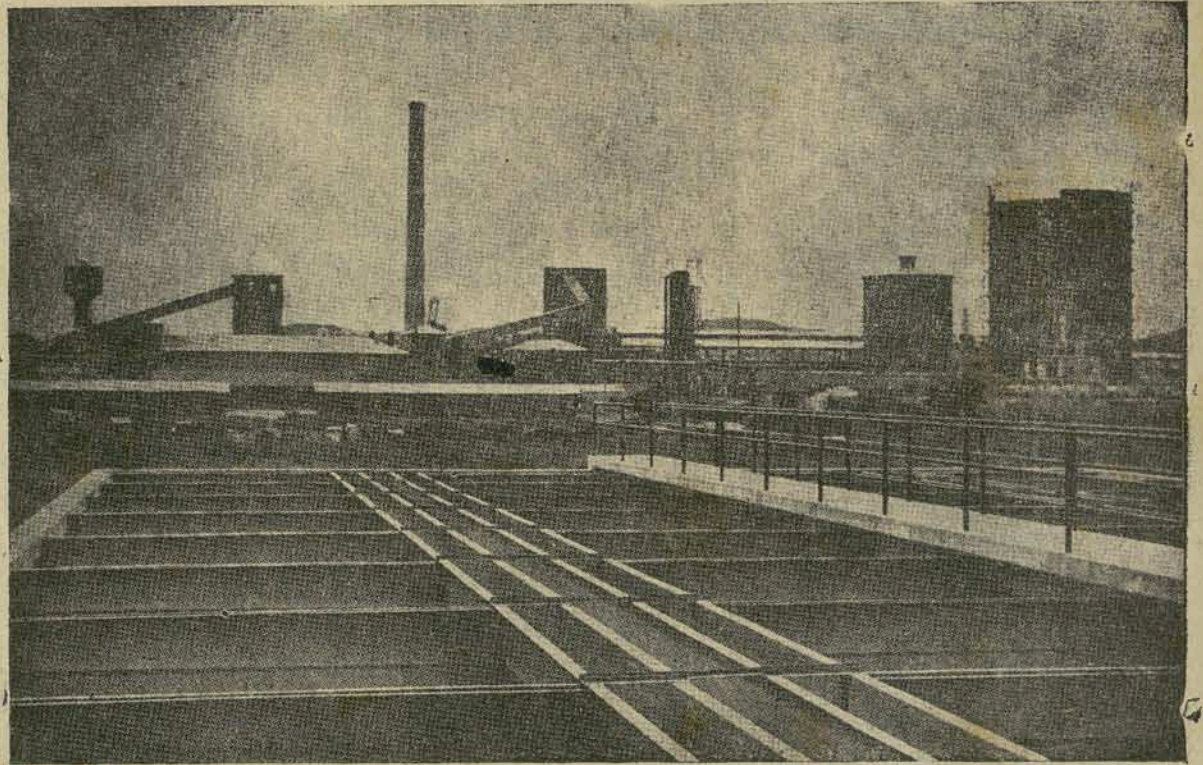
VOLTA REDONDA. — ABASTECIMENTO D'AGUA. Vista parcial da estação de tratamento d'água, aparecendo os tanques de decantação. Volta Redonda consumirá 1,7 vezes mais água do que o Rio de Janeiro, cabendo às necessidades do alto-forno a maior parcela.
