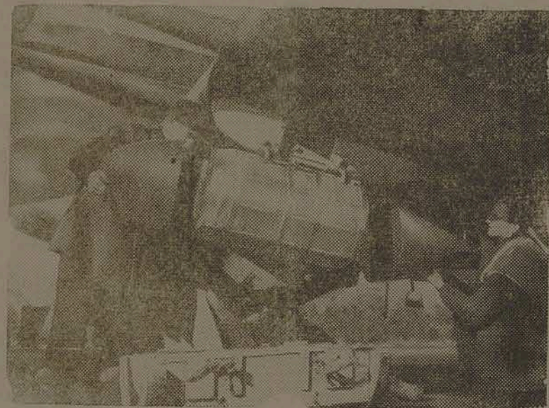
Caças bombardeiros Typhoon da 2ª Força Aérea Tática da RAF são carregados com um novo tipo de bombas, que ao explodirem não provocam crateras, tão prejudiciais ao avanço das tropas de terra. (B.N.S.).
