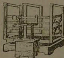
MODELO 3525 BALANÇA PARA PESAR SUINOS Armação em peroba rosa reforçada com ferro e aço temperado.
