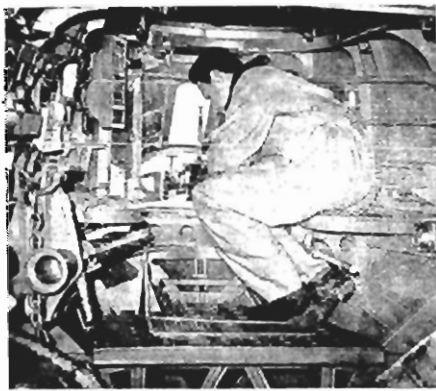
Conhecidos como os "encouraçados do ar", os "Sunderlands", hidroplanos poderosamente armados do Comando Costeiro, patrulham as proximidades e mesmo grandes distâncias além das costas britânicas. O lançador de bombas, na parte dianteira do aparelho, faz a pontaria com sua bomba, enquanto o "Sunderland" se afasta do comboio, afim de verificar um barco suspeito. (Foto de "British News Service").
