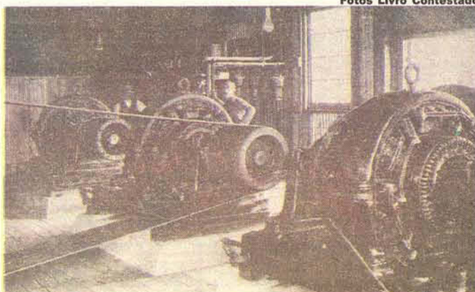
O alto grau de mecanização da serraria Lumber demandava a operação constante de grandes geradores em Três Barras
