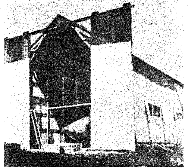
O primeiro hangar do mundo, Santos-Dumont construiu-o em Saint-Cloud no ano de 1889. Apresentava 7 metros de largura com 11 metros de altura e 30 metros de comprimento.
