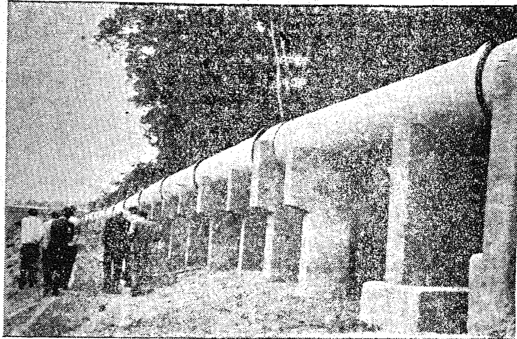
Estes tubos, com diâmetro de 800 mm, numa extensão de 1.300 metros, formam a adutora de água bruta, obra inteiramente concluída, que transporta água do rio à Estação de tratamento.
