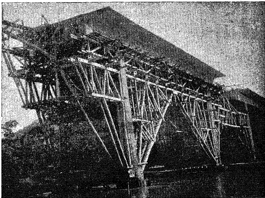
Adiantada fase da construção da Ponte Adolfo Konder, que hoje se inaugura.
