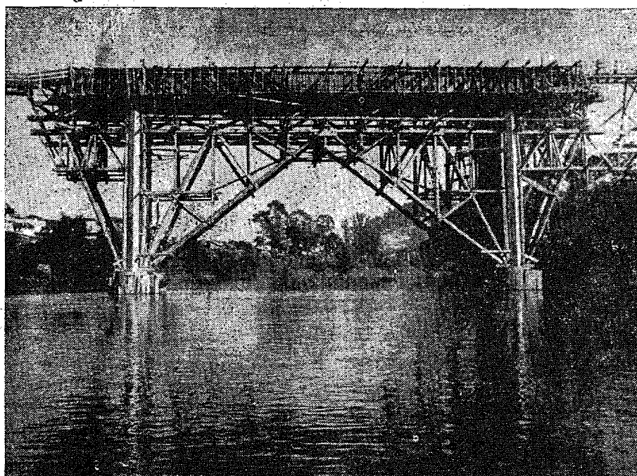
Flagrante colhido quando a imponente construção de concreto armado erguia-se sobre o Itajaí estendendo-se ás duas margens.
