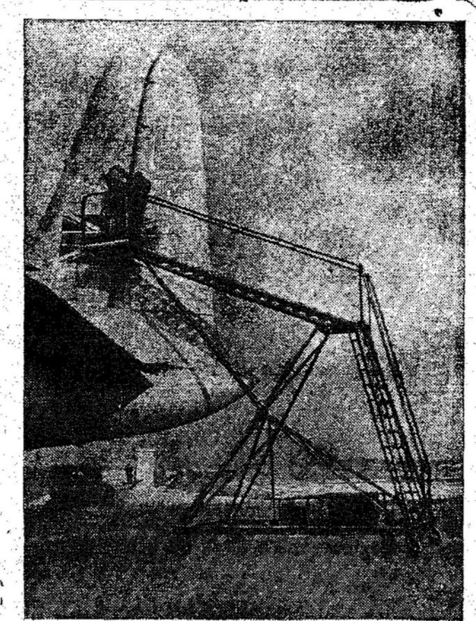
Uma versátil escada de trabalho, denominada "Girafa", ajuda a equipe de conservação dos aeroportos a atingir qualquer parte de um avião. Esta escada, fabricada por uma firma de Londres, pode carregar 4 homens a qualquer altura ou campo de trabalho necessário ao grupo de conservação. Na foto B. N. S. a "Girafa".
