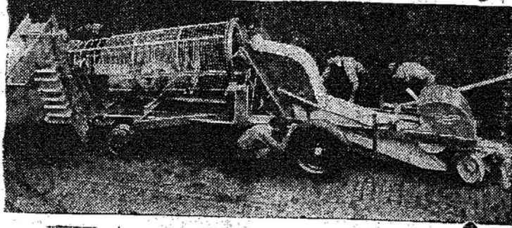
A curiosa máquina que se vê acima, construída numa fábrica de Londres, é um colhedor de batatas. Manobrada por um só homem, pode colher 1 1/2 hectare de batatas por dia. Em atenção ao pedido que a máquina fi-
