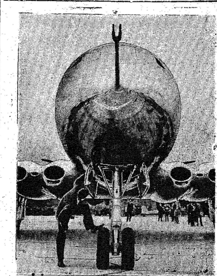
AVIAO DE TRANSPORTE A JATO — O primeiro grande avião de transporte britânico, provido de quatro motores a jato, "de Havilland Comet", recentemente passou por uma série de provas de terra e fez um voo de experiência. Catorze, destes aviões estão sendo construídos para serem usados nas grandes linhas aéreas internacionais da British Overseas Airways e a British European Airways e espera-se que estejam em serviço até 1952. Impulsionados por quatro motores "Ghost", embutidos nas asas e desenvolvendo uma empuxo de mais de 20.000 cavalos, o "Comet" está destinado a transportar 36 passageiros a 40.000 pés de altura a uma velocidade próxima das 500 milhas por hora. Vemos na fotografia o primeiro grande avião de transporte com quatro motores a jato. (Foto BNS).
