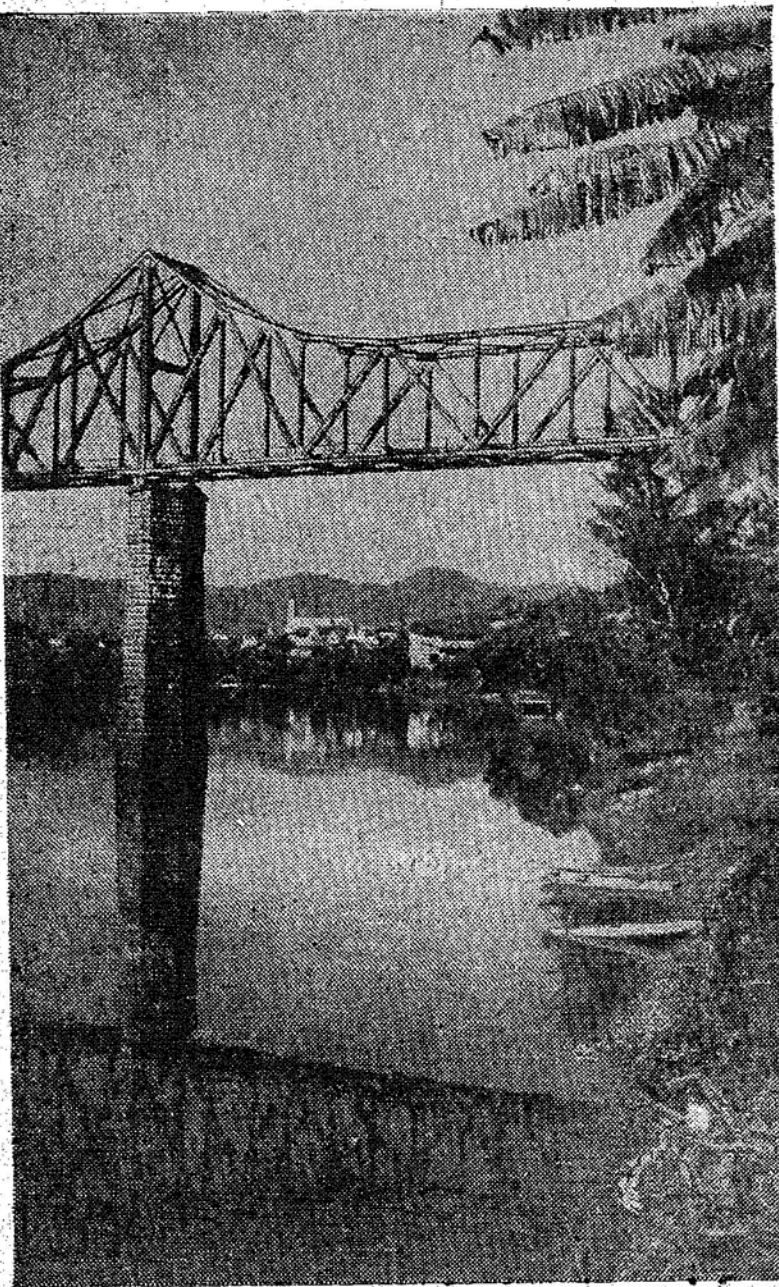
Trecho da ponte da Estrada de Ferro Santa Catarina, que atravessa o Itajaí-Açu. Pelo clichê, pode-se verificar o perigo de uma queda do pavimento
