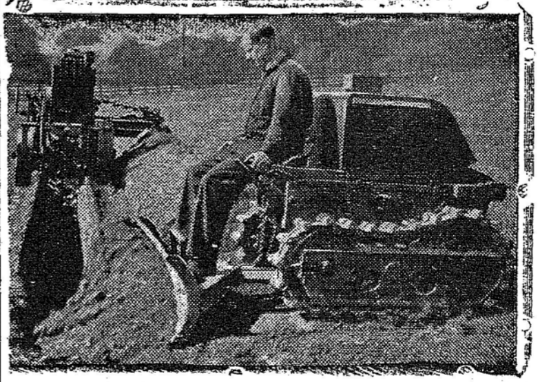
A MANUFATURA BRITANICA DE EQUIPAMENTO DE CONSTRUÇÃO — Esta maquina de fabricaçao britânica denominada "Caldorzer", serve para encher sulcos no terreno após a colocação de canos d'agua para abastecimento ou irrigação; realiza um trabalho igual ao de 10 homens — (BNS).
