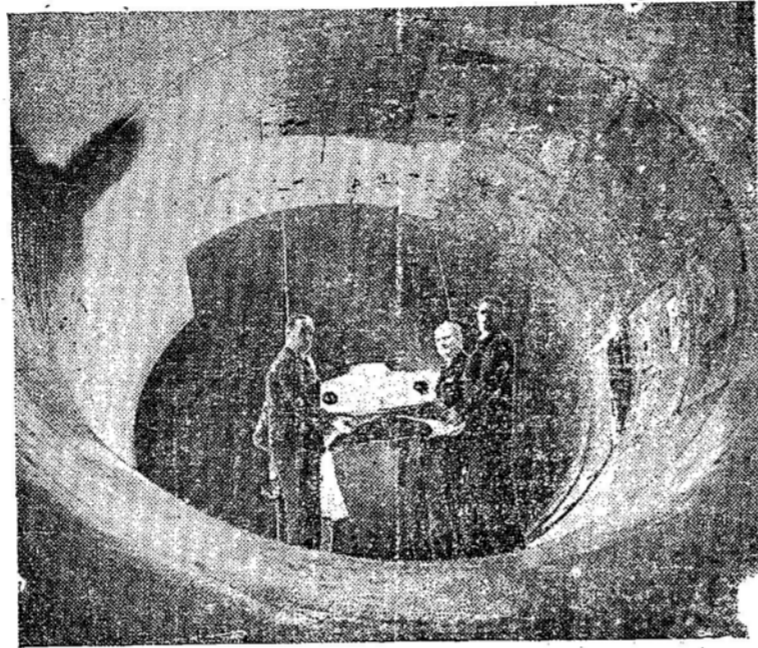
Sir Malcolm Campbell pretende bater seu próprio recorde de velocidade sobre a agua, 141,74 milhas por hora, em lancha de propulsão a jato. A fotografia mostra-nos Sir Malcolm com funcionarios da Fairey Aviation Company fazendo experiências com um modelo da lancha, denominada "Bluebird" (Passaro Azul) no tunel de provas daquela fabrica de motores de avião. (B.N.S.)
